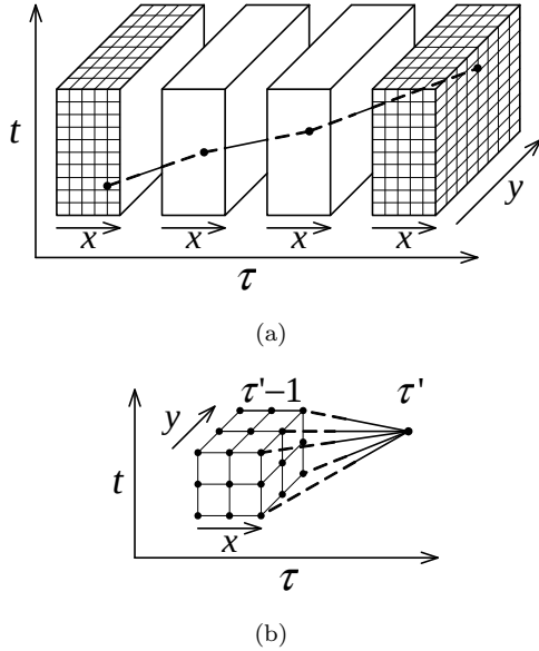
図 4 DP マッチングの概要図. (a) 計算空間は 4 次元で表現される. (b) DP パス：局所的に最適な経路が 27 経路から選択される。
