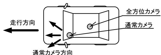
図 6 カメラの取り付け位置．
