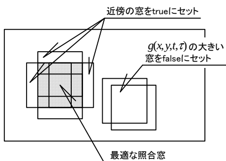
(b) 照合範囲の制限．
