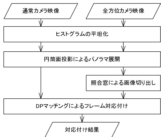
図 1 フレーム間対応付け処理の流れ．
