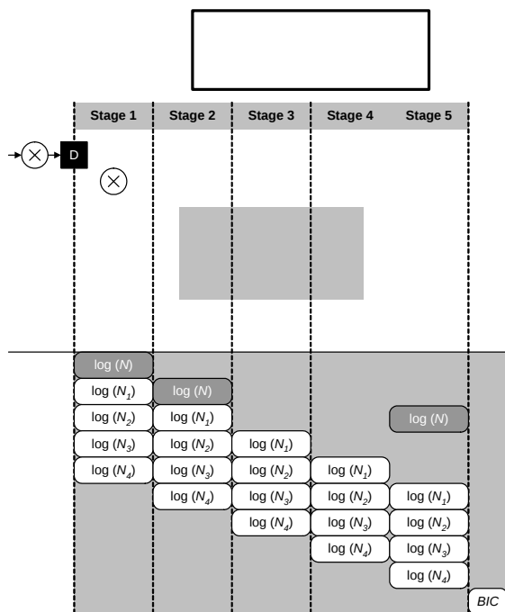
図 3 ベイズ情報量規準処理装置の構造図. 内部には 5 段階にわたるパイプラインがある.
