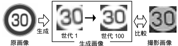
Fig. 2 Parameter estimation process
