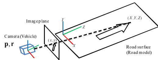
図5: 道路モデルと車両モデル
