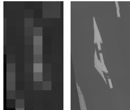
(b) 約 60cm/pixel : (左) 空撮画像 (右) 道路画像地図構築結果
